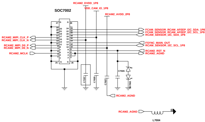
RCAM2_2M_Macro_24pin
