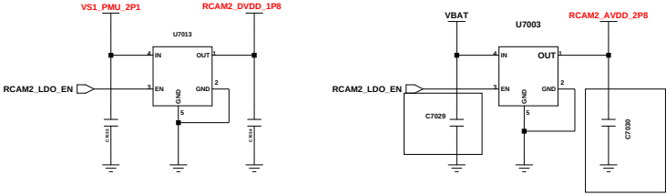
RCAM2_LDO
